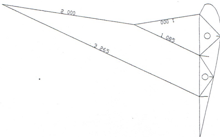
Caissons n° 2 & 8
