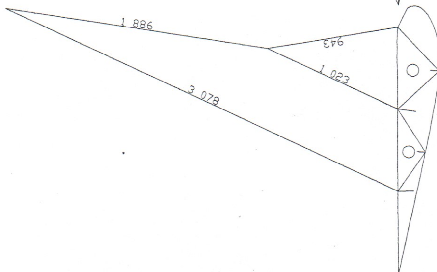
Caissons n° 2 & 8
